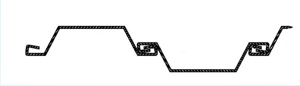
চিত্র-১১ স্টীল শিট পাইল
