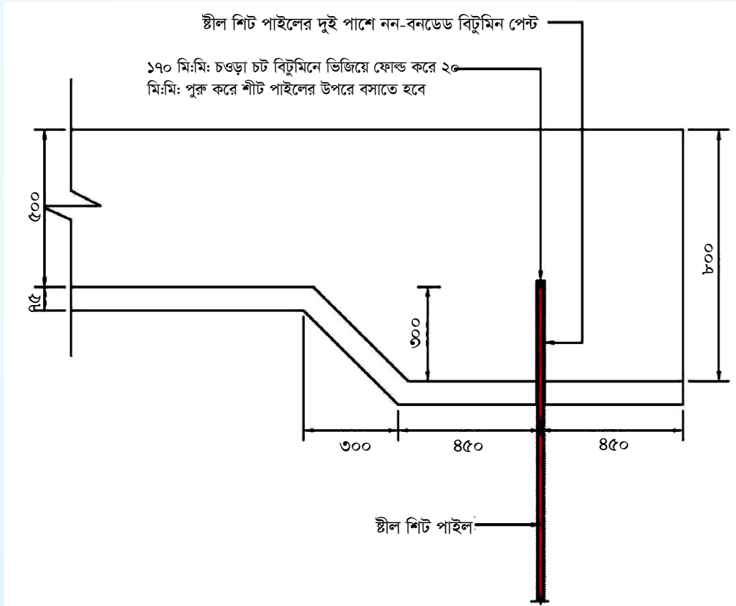
চিত্র-১২ ফ্লোর স্লাবের সাথে স্টীল শীট পাইলের এংকর ও কুশন ব্যবস্থা
