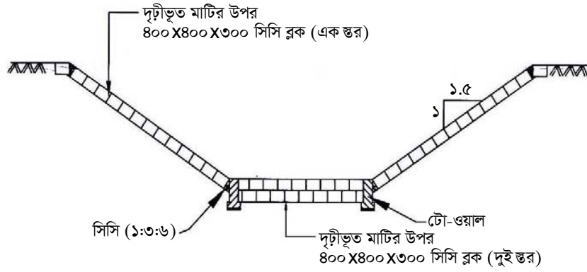
চিত্র-১০ লঞ্চিং এ্যাপ্রোনে ব্লক বসানো
