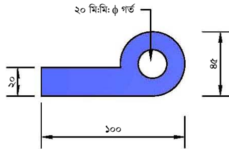
চিত্র-১৫ ফ্ল্যাপ গেইটের রাবার সীল (তুলনামূলক ভারি রাবার সীল)
